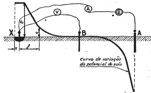
Figura 1 Medição da resistência de terra de um eléctrodo de terra «X»
